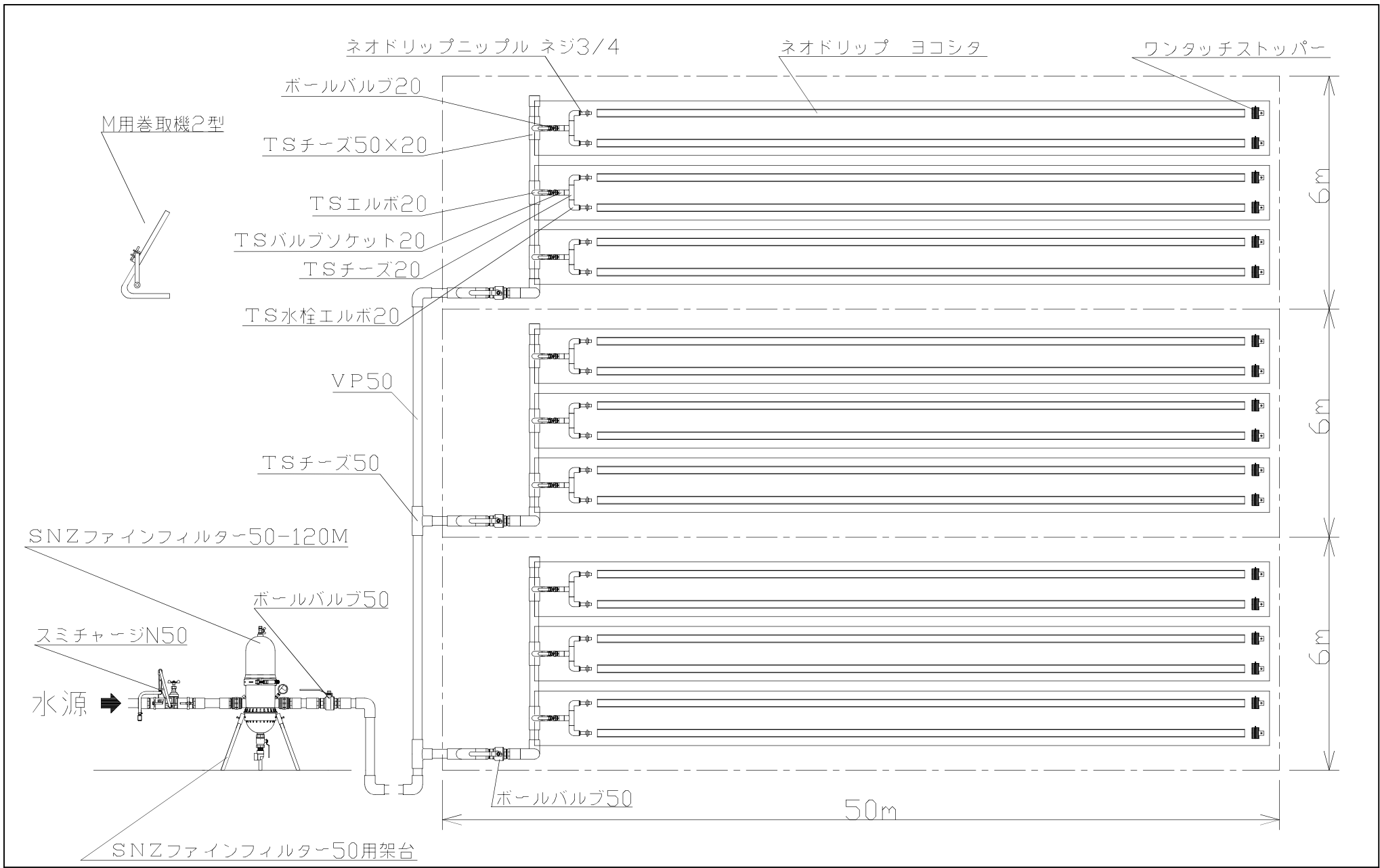
ネオドリッ ヨコシタ 配管例 (10a)
