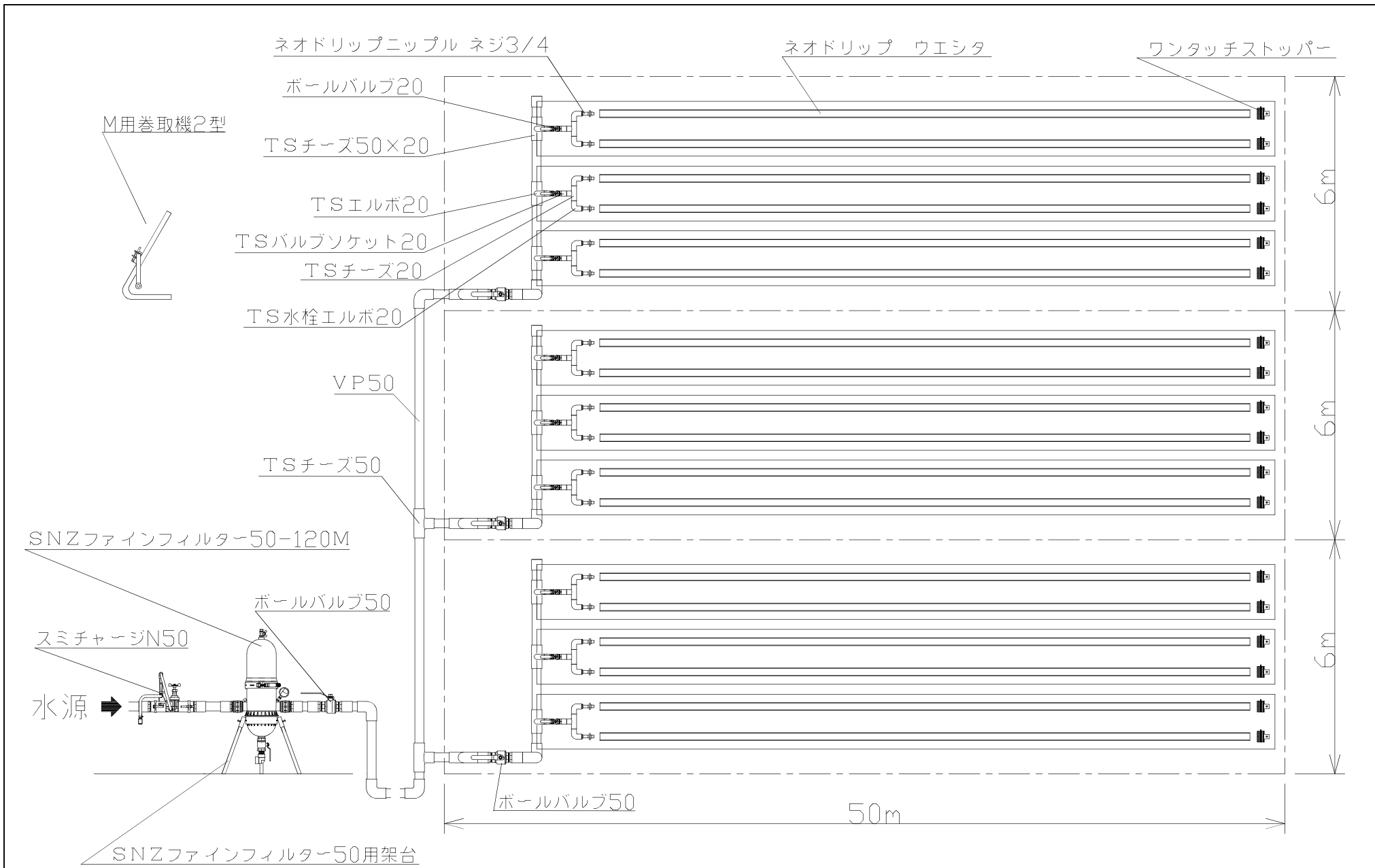
ネオドリッパー ウエシタ 配管例 (10a)
