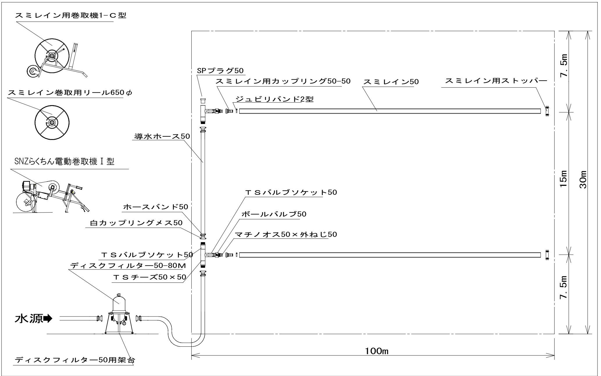
スミレイン50 配管例 (30a)
