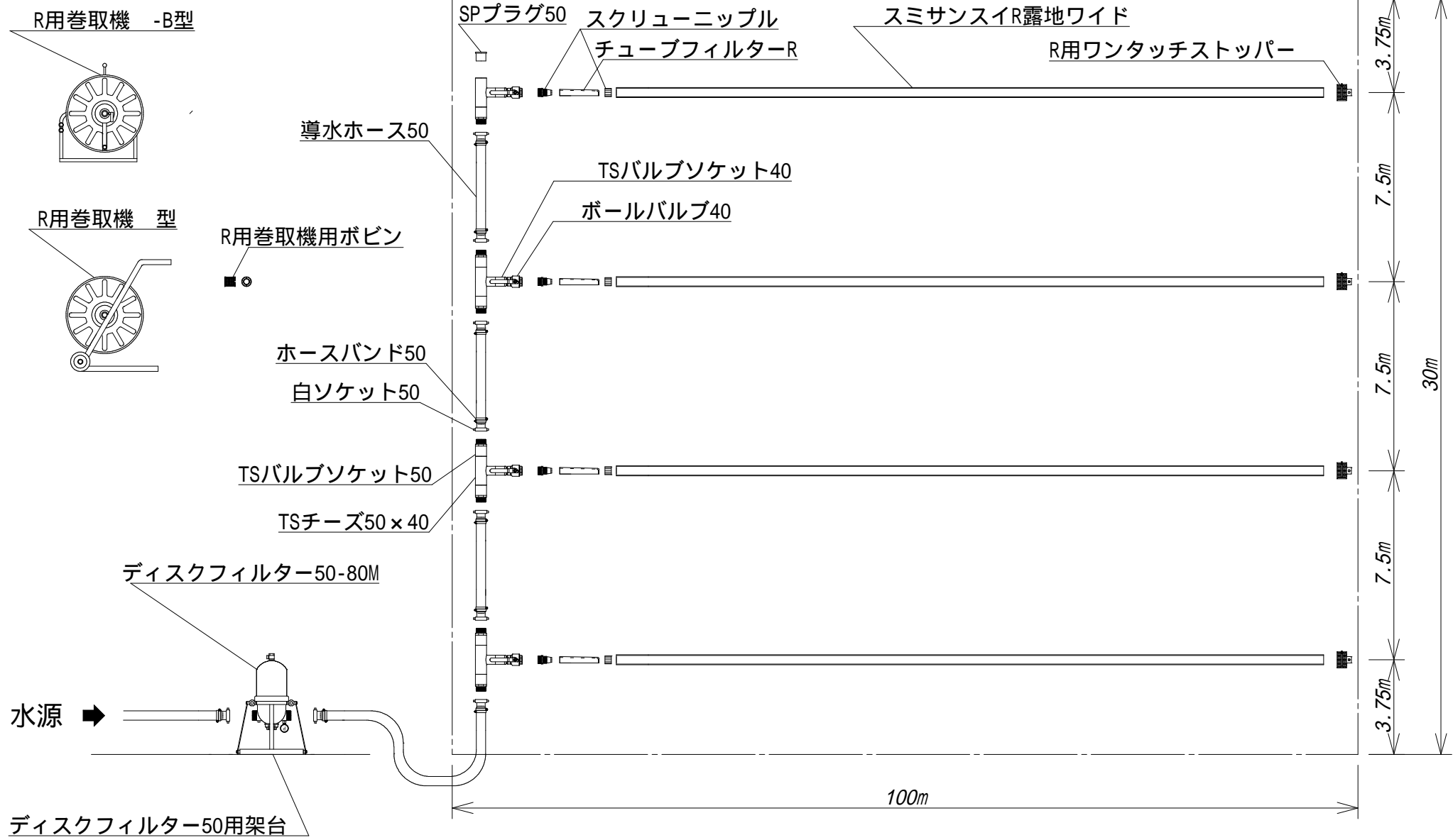
スミスンスイR露地ワイド 配管例 (30a)
