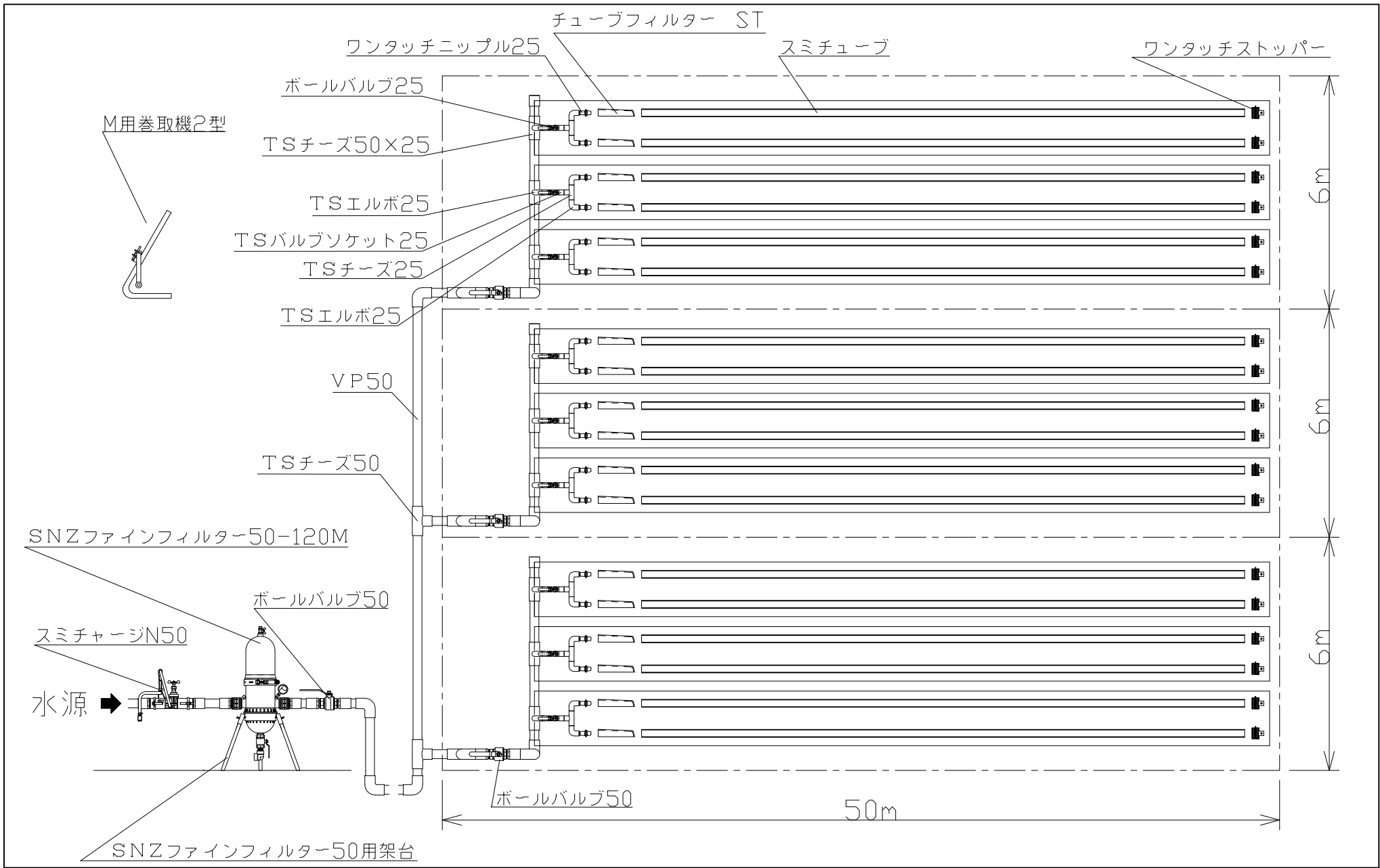
スミチューブ 06-60、06-120 配管例 (10a)
