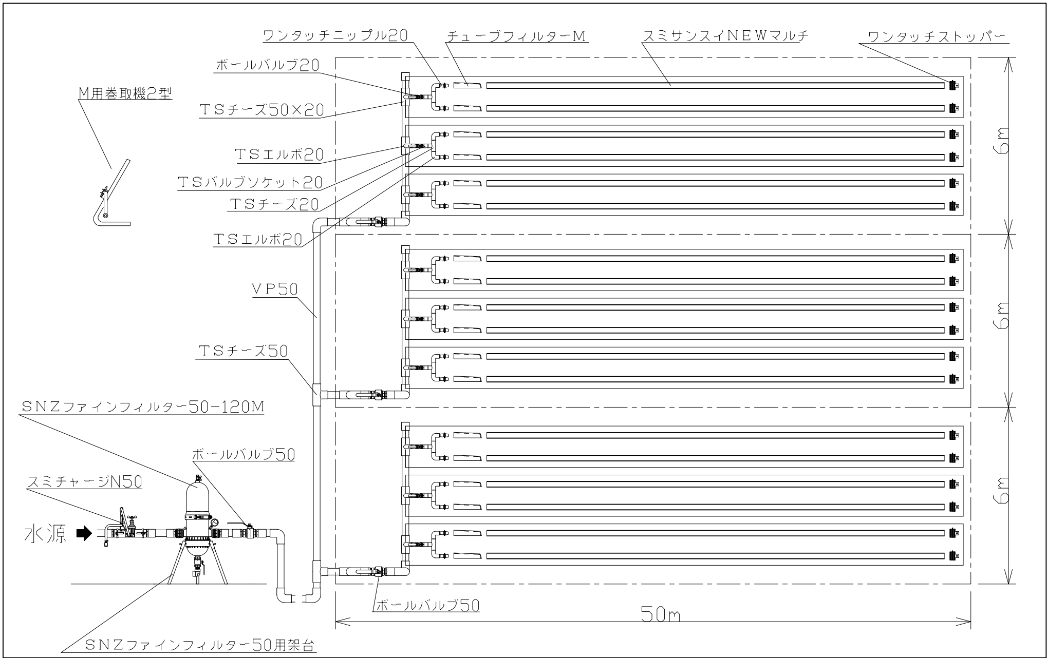
スミサンスイNEWマルチ 配管例(10a)
