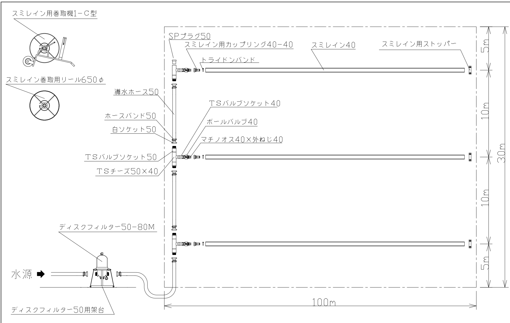
スミレイン40 配管例 (30a)
