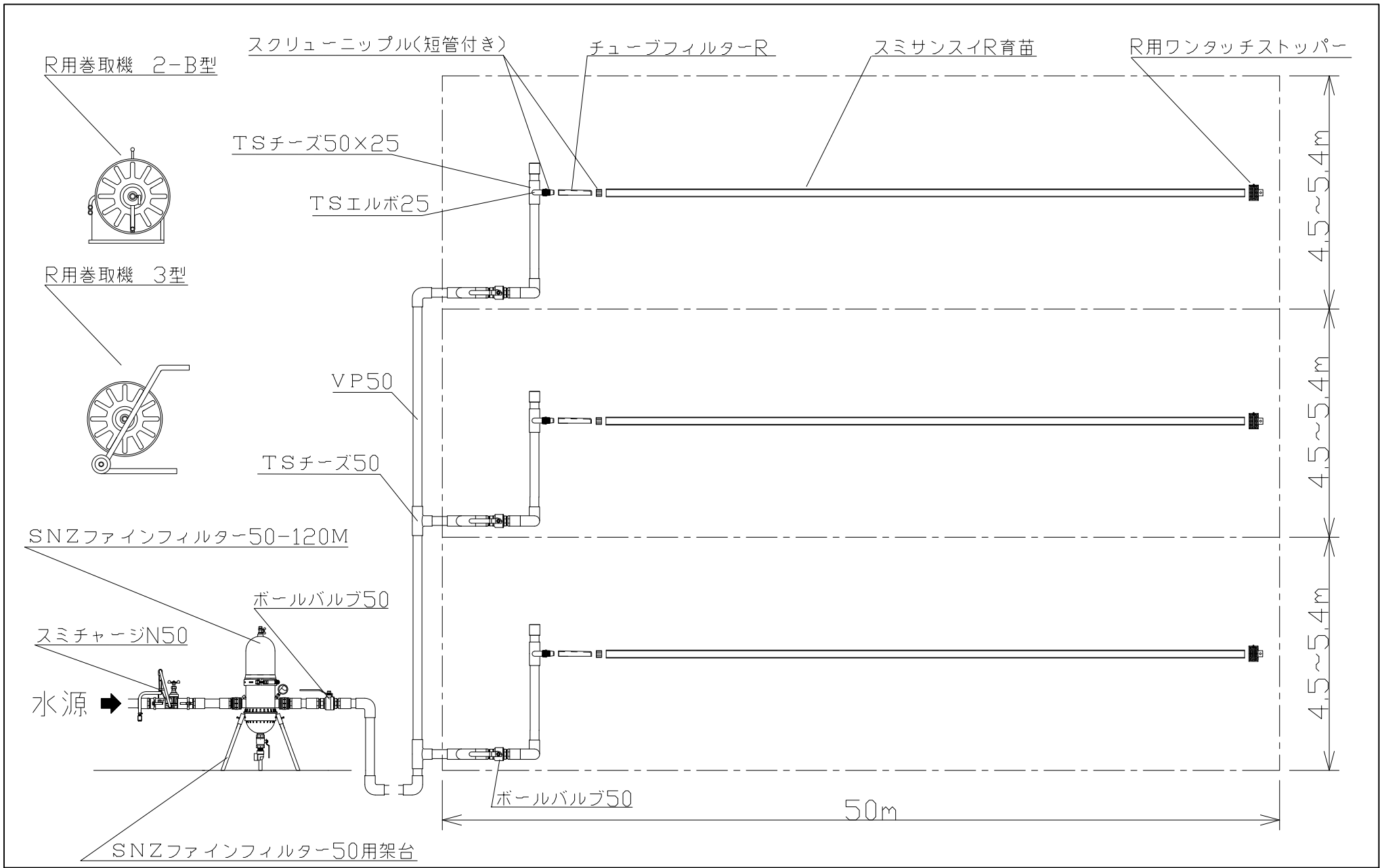
スミサンスイR育苗 配管例(10a)
