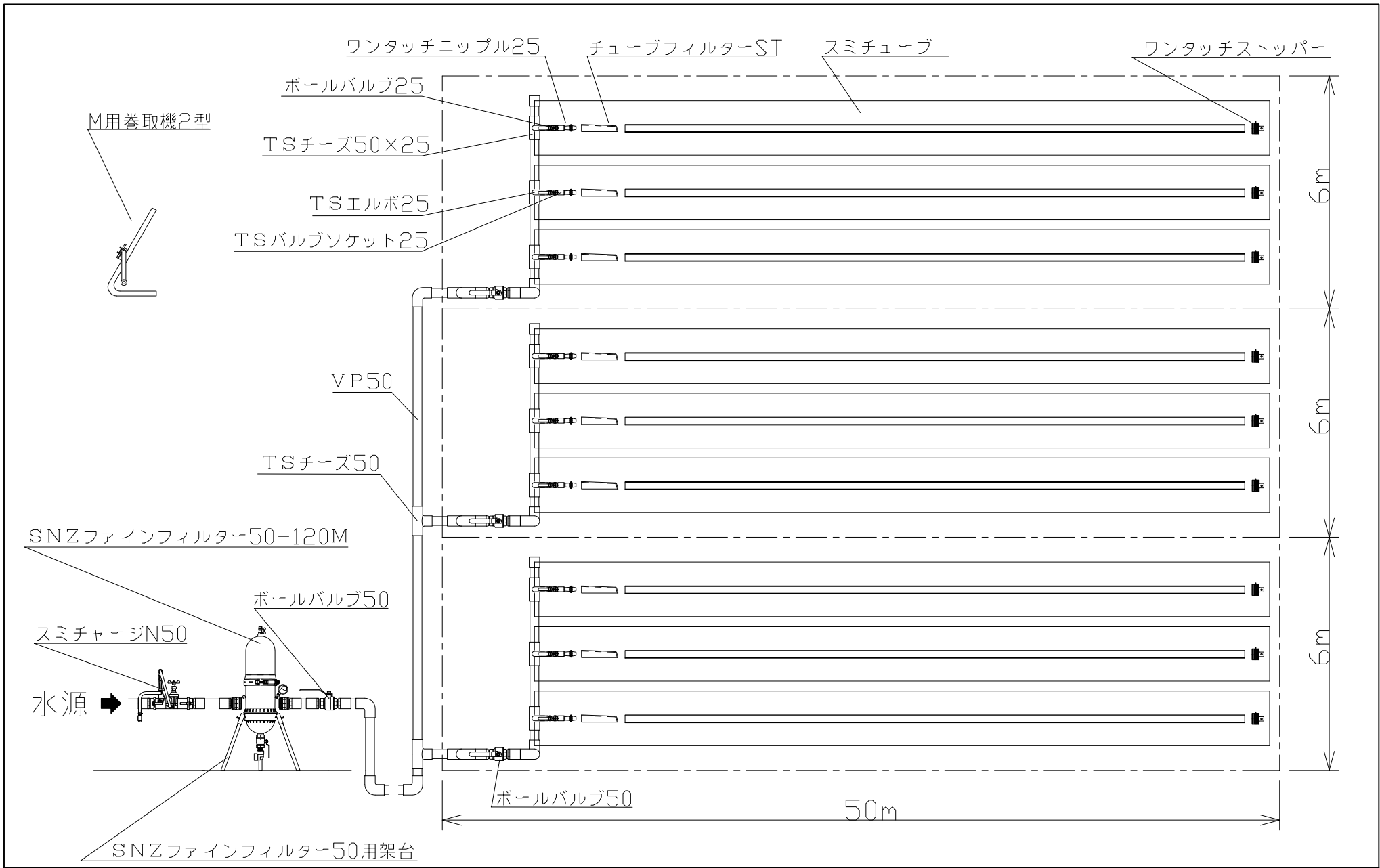
スミチューブ ウェシタ 配管例 (10a)
