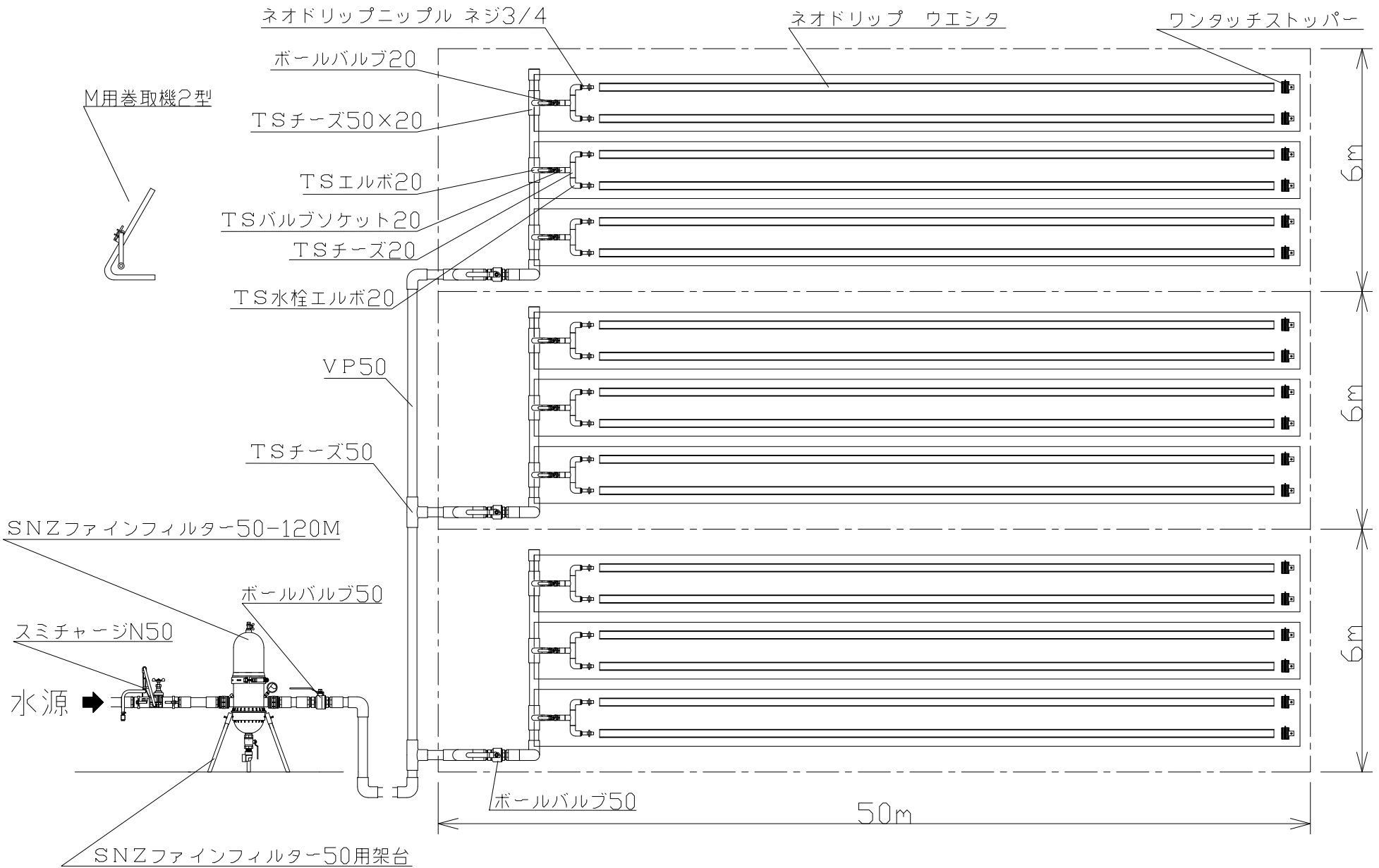
ネオドリップ ウエシタ 配管例 (10a)
